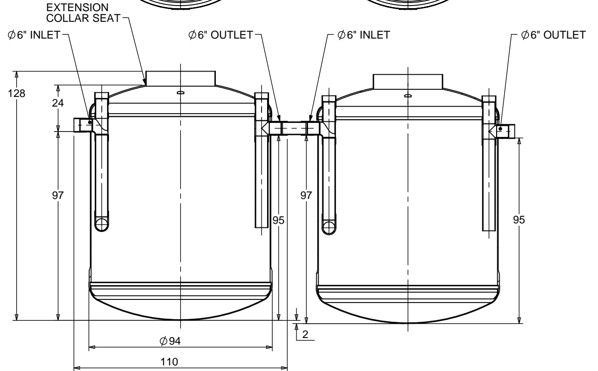
SECTION A-A
