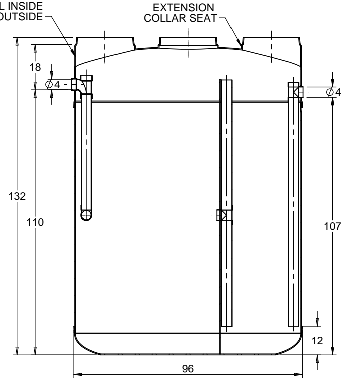
SECTION A-A SCALE 1 : 40
